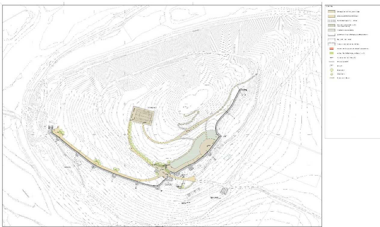
Το σχέδιο αναρτάται ευκρινέστερα στο φυσικό του μέγεθος με όνομα αρχείου F_ΧΡΥ Α09
